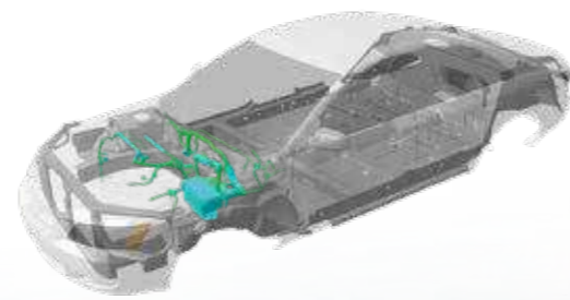
Dây điện điều khiển động cơ Wire harness - Control
