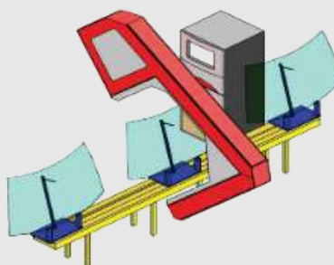
Thiết bị kiểm tra quang học kính chắn gió Optical inspection equipment for windshields
