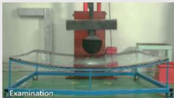
Máy đo độ bền cơ học Mechanical Strength Tester
