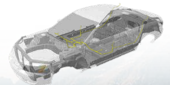
Dây điện túi khí Wire harness - Airbag
