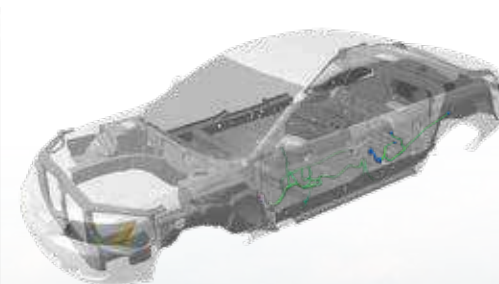
Dây điện cửa trước trái Wire harness - DR driver side
