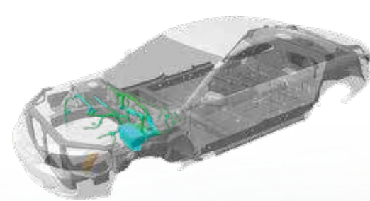
Dây điện điều khiển động cơ Wire harness - Control
