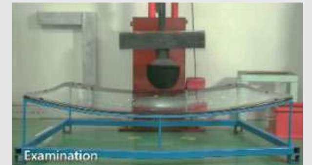
Máy đo độ bền cơ học Mechanical Strength Tester
