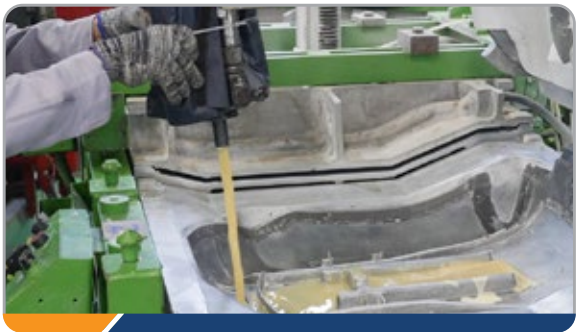
Công đoạn đổ hóa chất vào khuôn Pour chemicals into the mold
