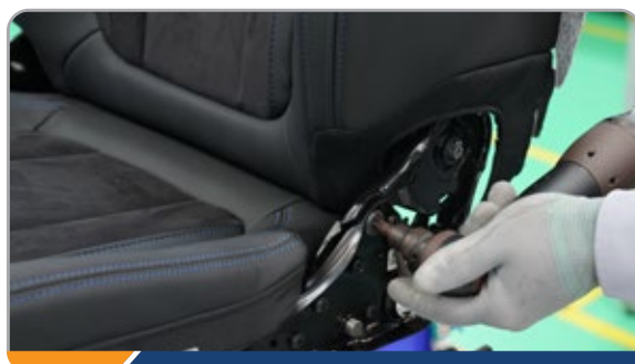
Siết lực và kiểm tra lực siết Tightening and torque testing
