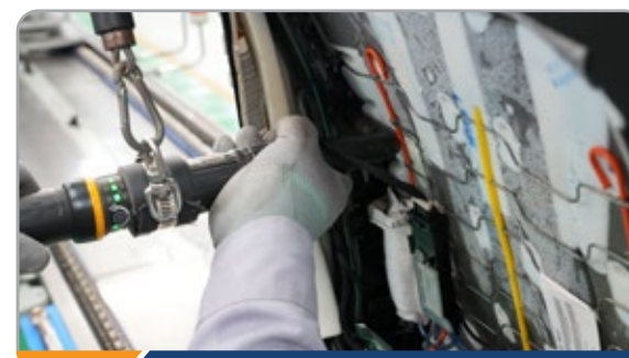
Lắp túi khí Airbag assembly
