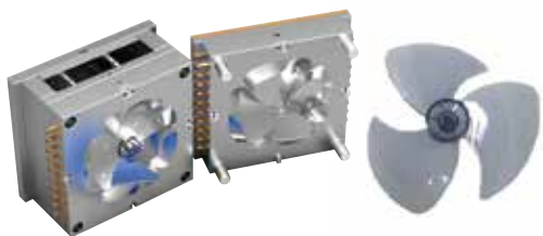
Khuôn cánh quạt nhựa Plastic propeller of fan Mold
