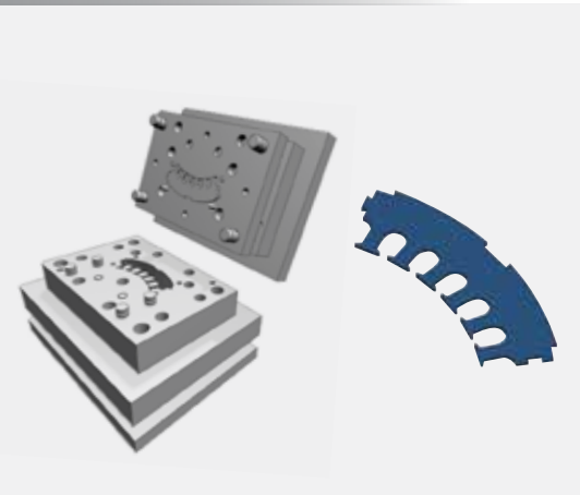
Khuôn dập Chi tiết phe stator Lamination stator Stamping Die
