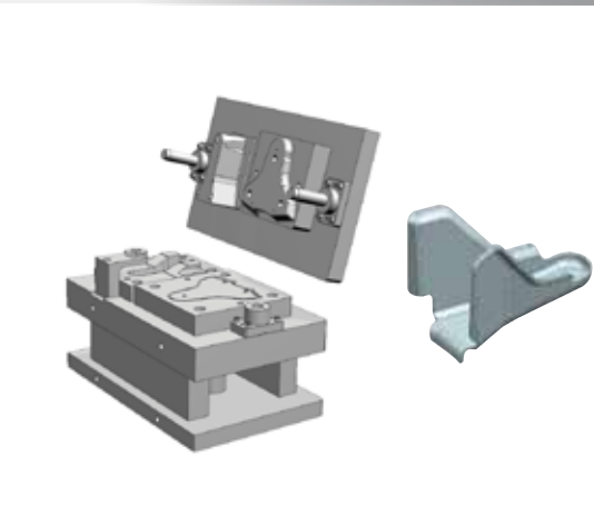
Khuôn dập chi tiết treo ống xả Exhaust system component Stamping Die
