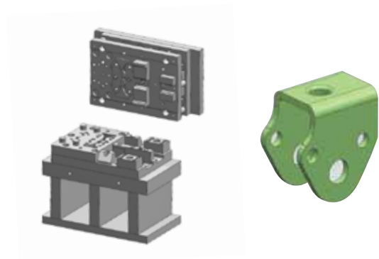
Khuôn liên hợp xả cuộn U cần lật ty Element (U - Shape) Progressive Die
