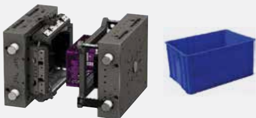
Khuôn rổ nhựa Plastic Basket Mold
