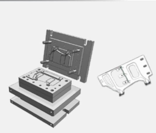
Khuôn dập bách bắt dây điện khóa an toàn trái Wiring hold part for LH safety locker Stamping Die
