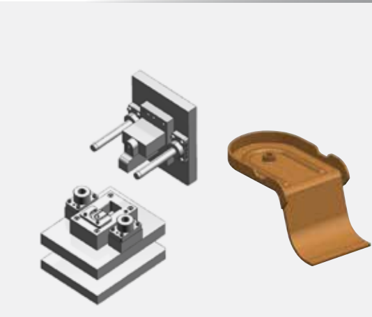
Khuôn dập biên dạng chi tiết bách ghế giữa Plate BRKT FRM back FRT CTR Stamping Die
