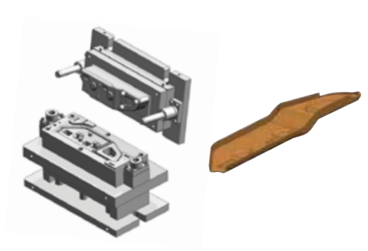
Khuôn dập chi tiết bách ghế tài Plate BRKT FRM back FRT LH Stamping Die
